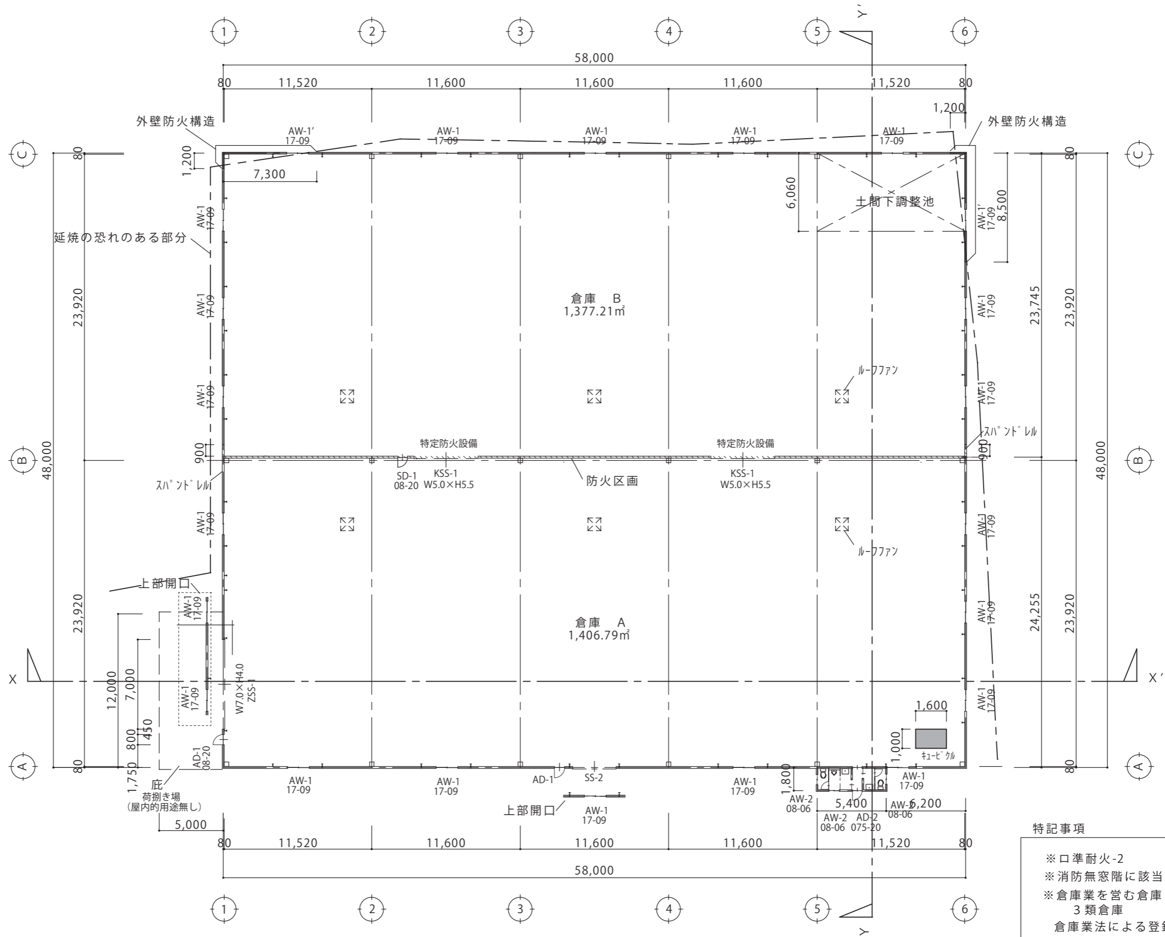
(株)平中サービス笠原倉庫 平面図
